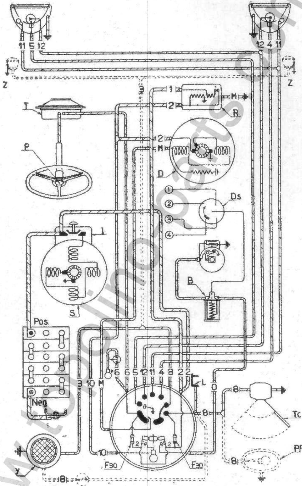
Abb. 6. — Schaltschema der elektrischen Anlage.
